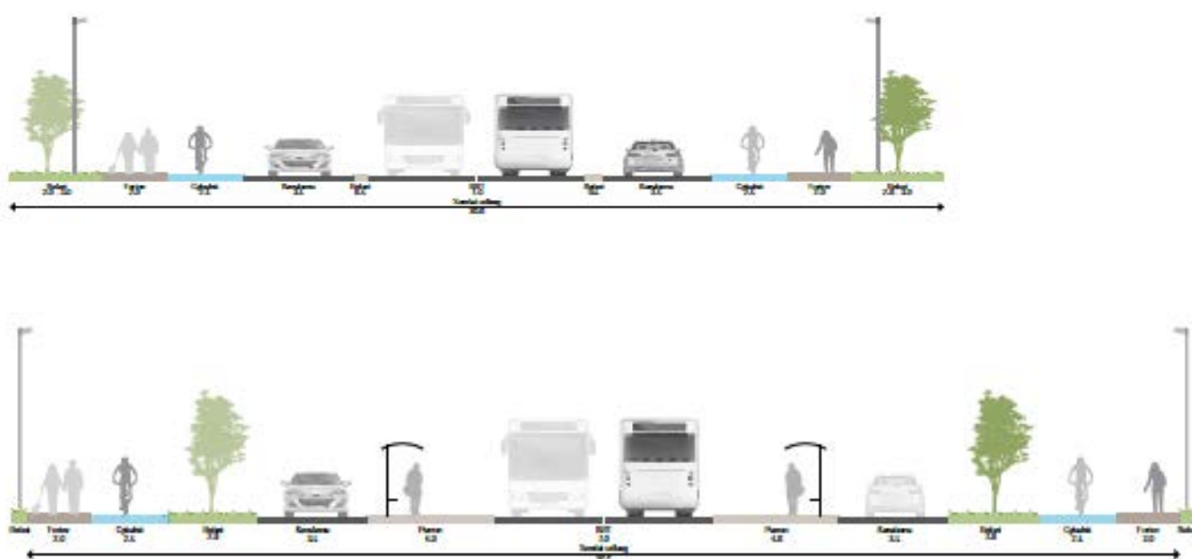
Figur 21 Mulige tværsnit på Tårnvej hhv. nord for Rødovre Parkvej og ved Rødovre Centrum, hvis en vognbane for biltrafik inddrages til begrønning og bredere stier.
