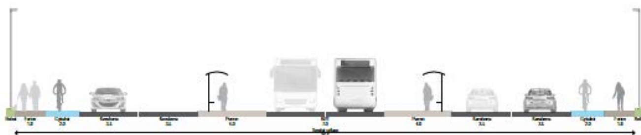
Figur 16 Standard station med midterlagt BRT-tracé og standard bredde på platforme og vejbaner, brugt i tracé-gennemgangen og optegningen. I den nærmere detaljering vil det være muligt at justere bredder, herunder kan bredde på køresporene ved stationerne reduceres til min. 3 m, da bussernes hastighed er lav ved stationerne og da busserne skal helt ind til kantstenene for at udveksle passagerer.
